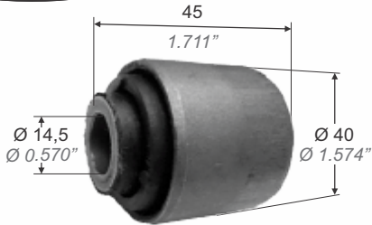
BUJE BIELETA TENSORA (CORTO) TENSILE BAR BUSHING (SHORT)
